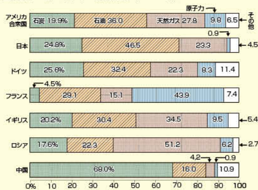
主要国の一次エネルギー供給構成（2012年）
